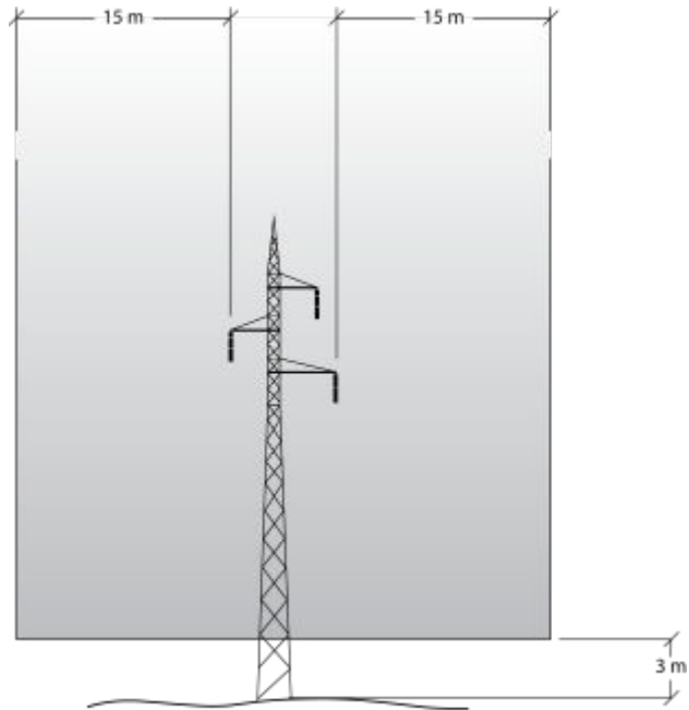
Figur 4 Højspændingsluftledninger 40-400 kV
