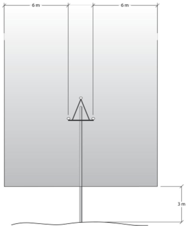
Figur 3 Højspændingsluftledninger 10-40 kV
